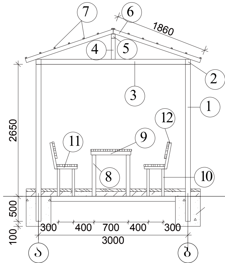
ჯრილი I-I
