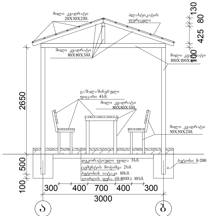
ჯრილი I-I
