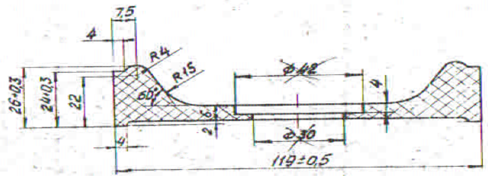
A-A M 1:1
