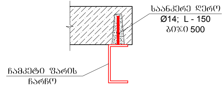
ჭრილი 1-1
