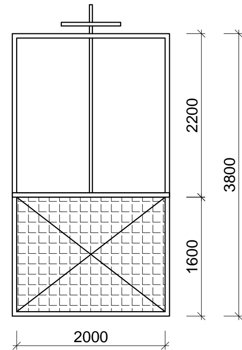
შემტბორავი ფარი მქანნიკური ამძრავით - ПС 200X160x380 (Серия 3.820.2-37 Затворы плоские поверхностные скользящие)
