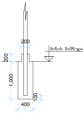
ჭრილი 1-1
