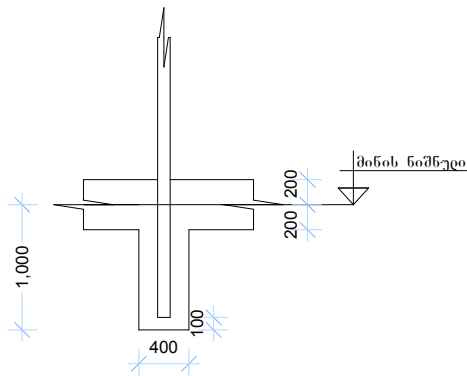
ჭრილი 2-2
