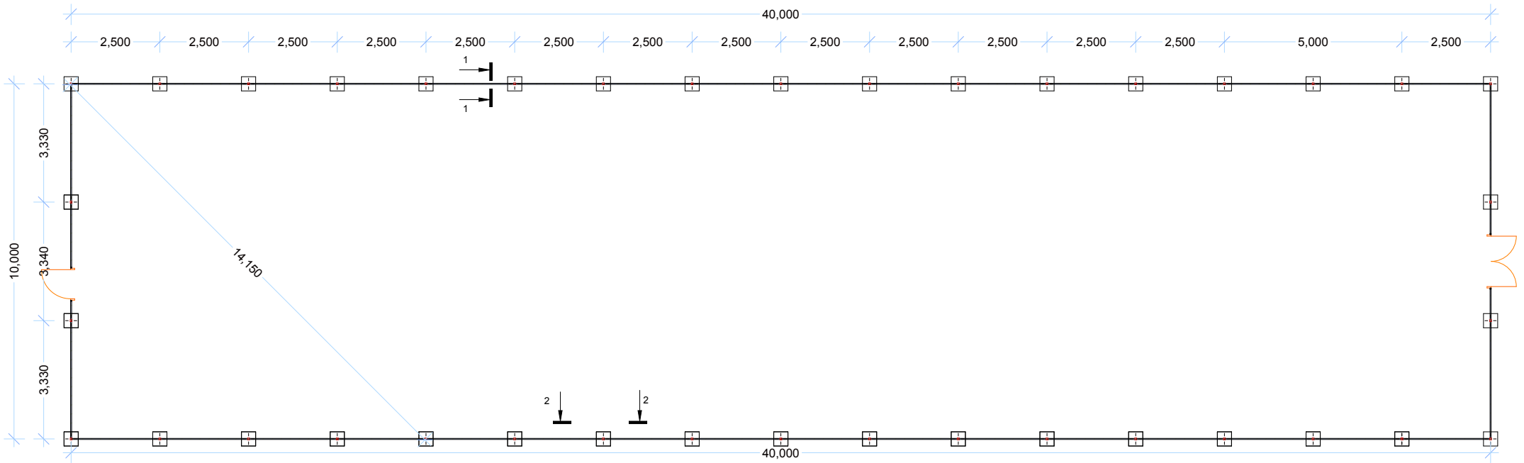
სათბურის გეგმა
