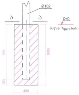
ჭრილი ა-ა
