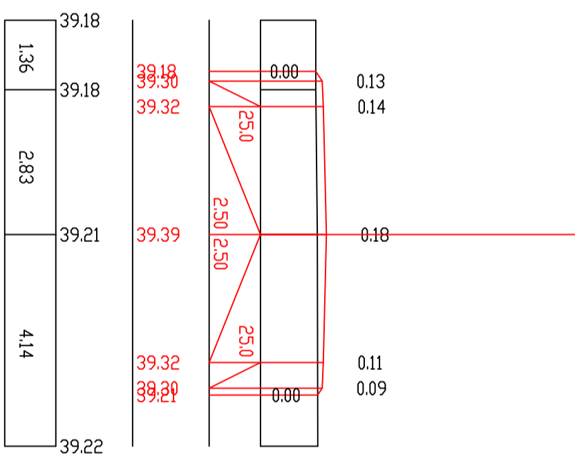
П-6 ПК 1+0,00
