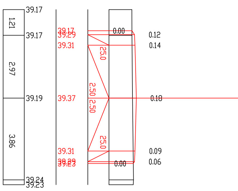
П-8 ПК 1+40,00
