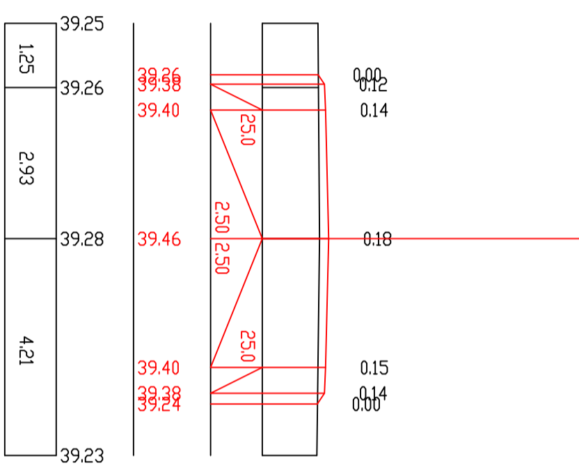
П-5 ПК 0+80,00
