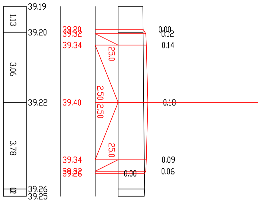
П-9 ПК 1+60,00
