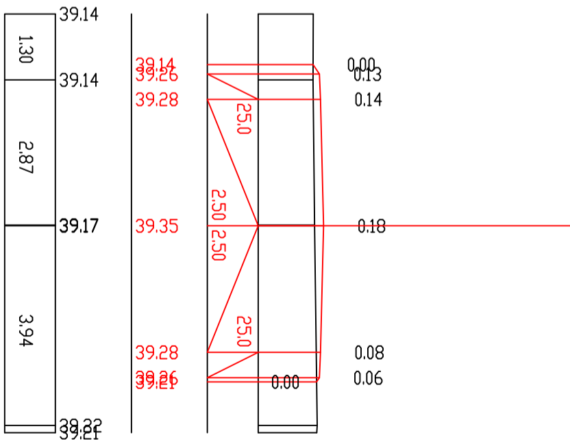
П-7 ПК 1+20,00
