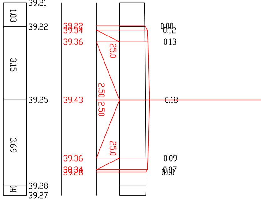
П-10 ПК 1+80,00
