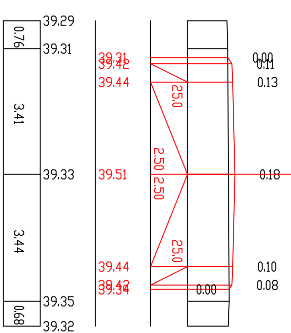
П-16 ПК 3+0,00
