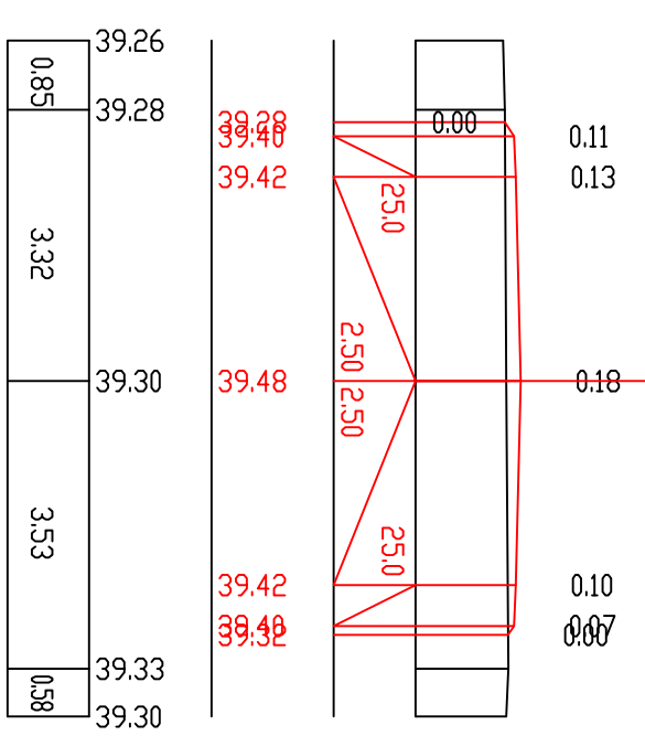
П-15 ПК 2+80,00
