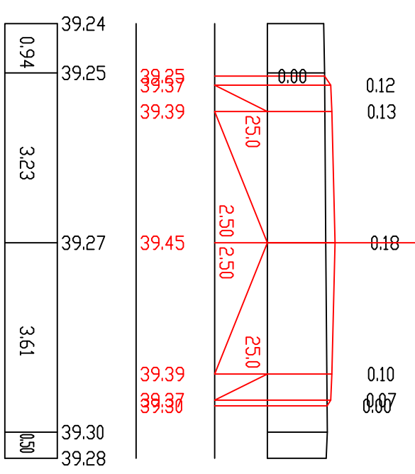
П-14 ПК 2+60,00
