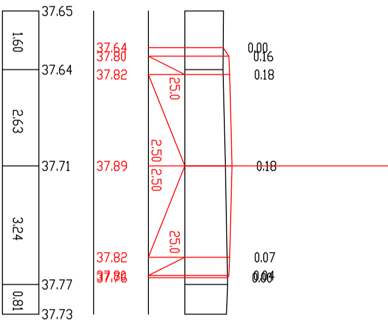
П-57 ПК 11+20.00
