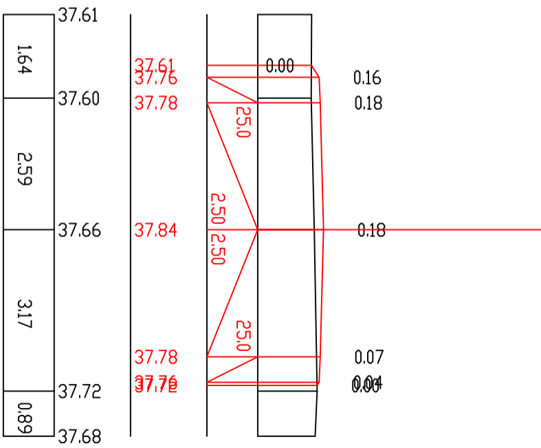
П-58 ПК 11+40.00
