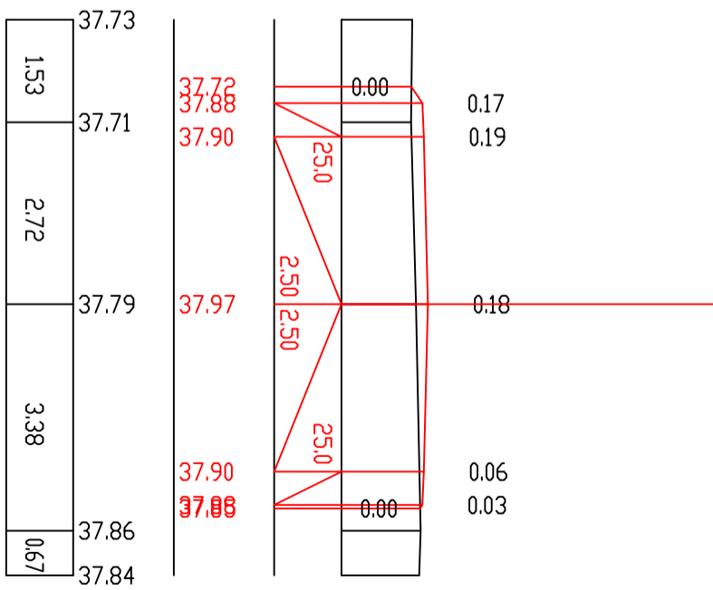
П-55 ПК 10+80.00
