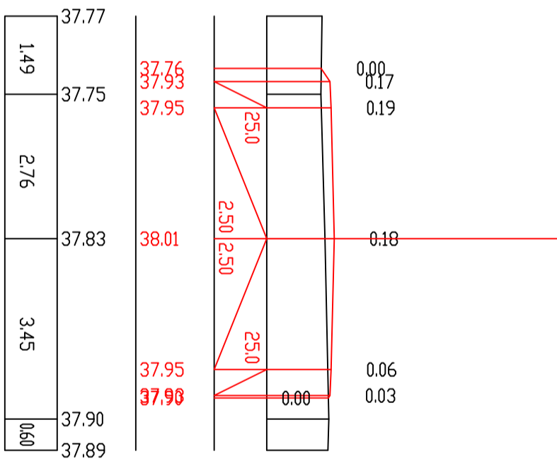
П-54 ПК 10+60.00
