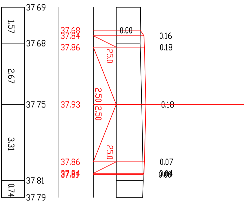
П-56 ПК 11+00.00
