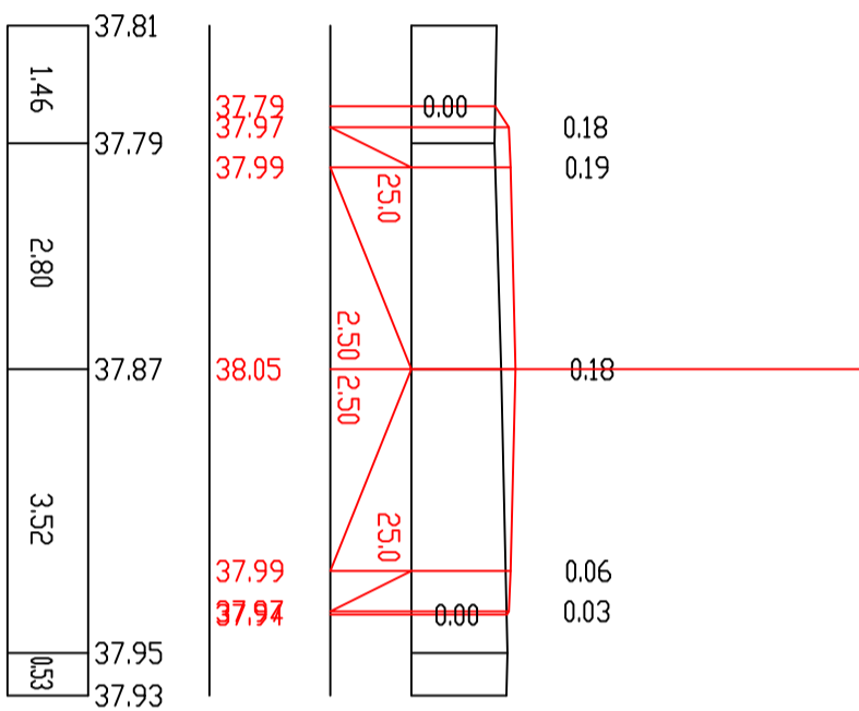
П-53 ПК 10+40.00
