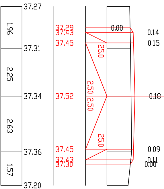
П-69 ПК 13+60,00
