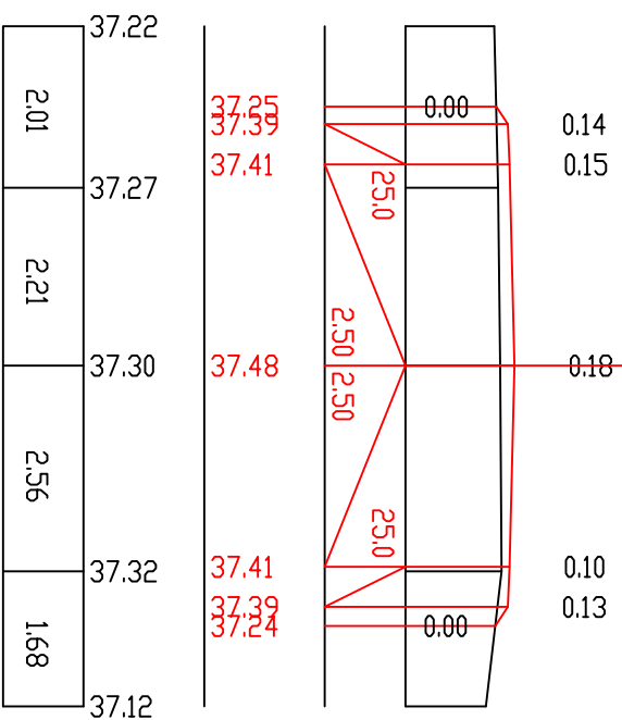
П-70 ПК 13+80,00
