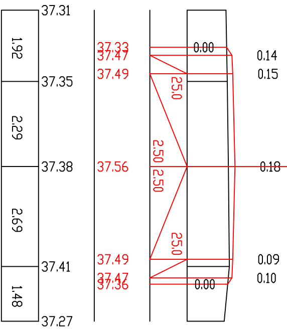
П-68 ПК 13+40,00
