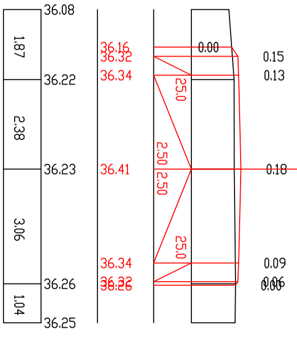
П-94 ПК 18+60,00
