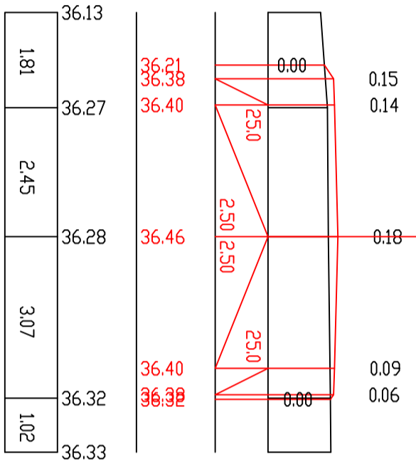
П-92 ПК 18+20,00
