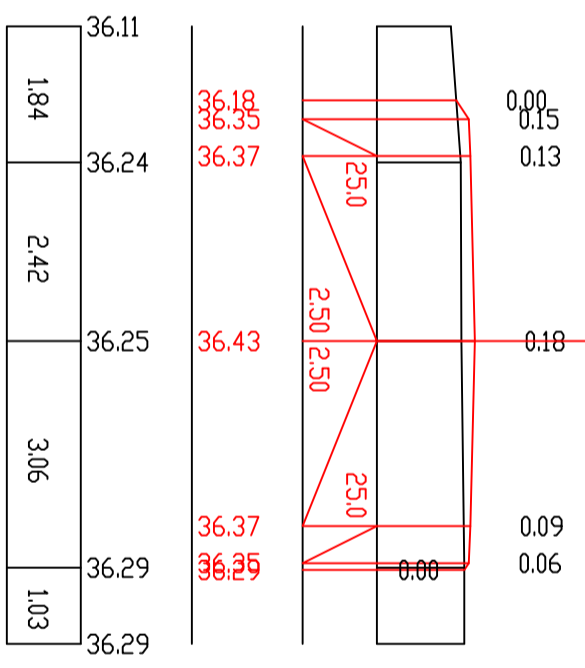
П-93 ПК 18+40,00
