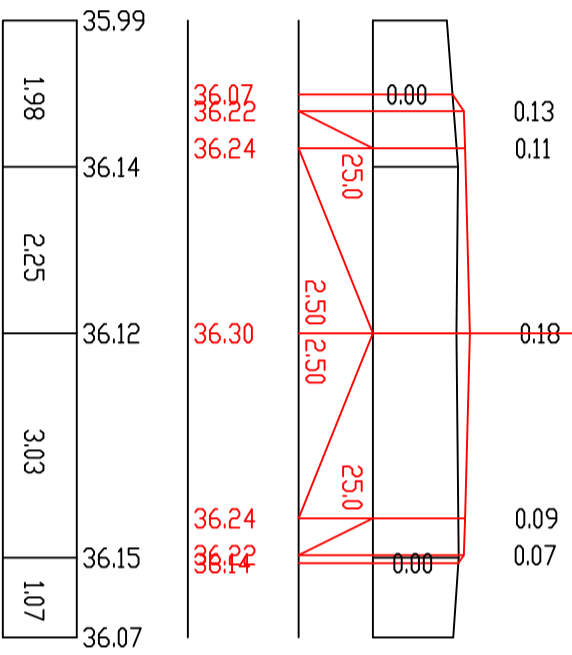
П-98 ПК 19+40,00
