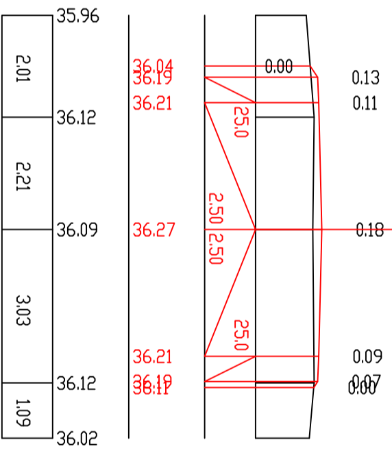
П-99 ПК 19+60,00
