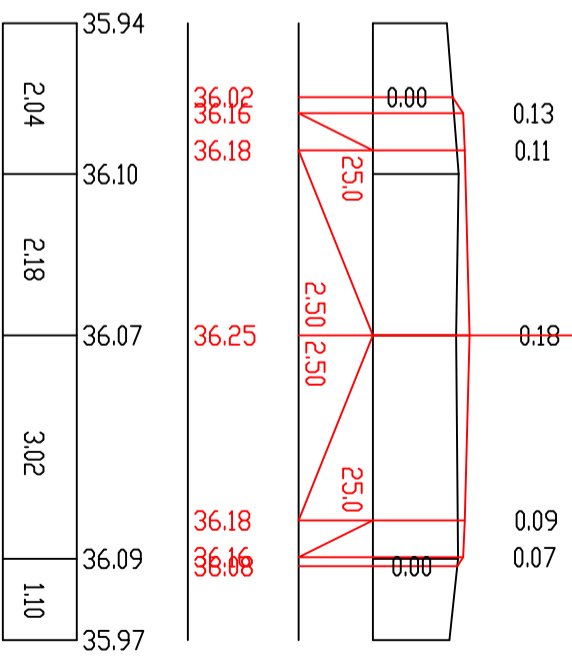
П-100 ПК 19+80,00
