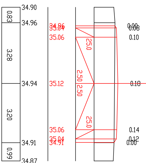
П-118 ПК 23+40,00
