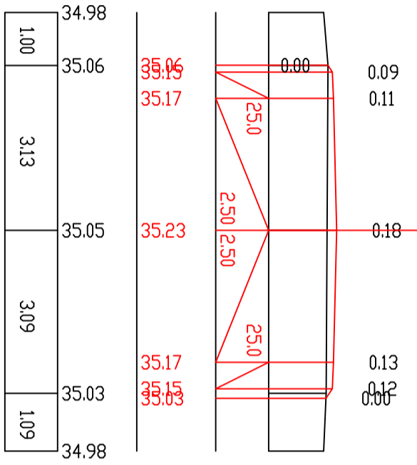
П-116 ПК 23+00,00
