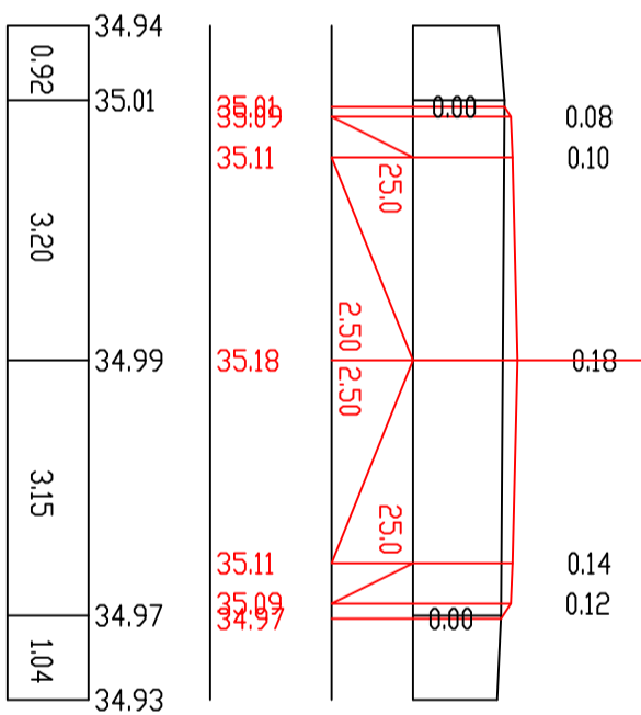
П-117 ПК 23+20,00
