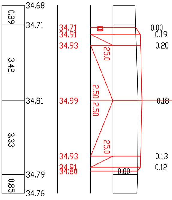
П-124 ПК 24+60.00
