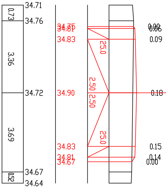
П-122 ПК 24+20.00
