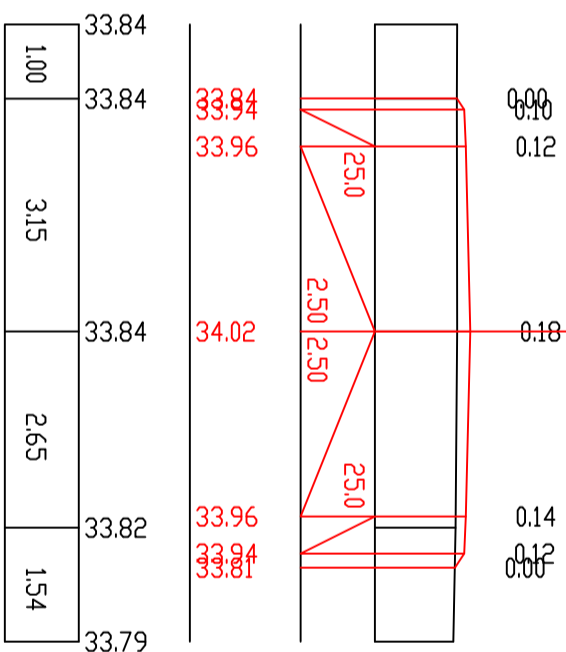
П-147 ПК 29+20.00
