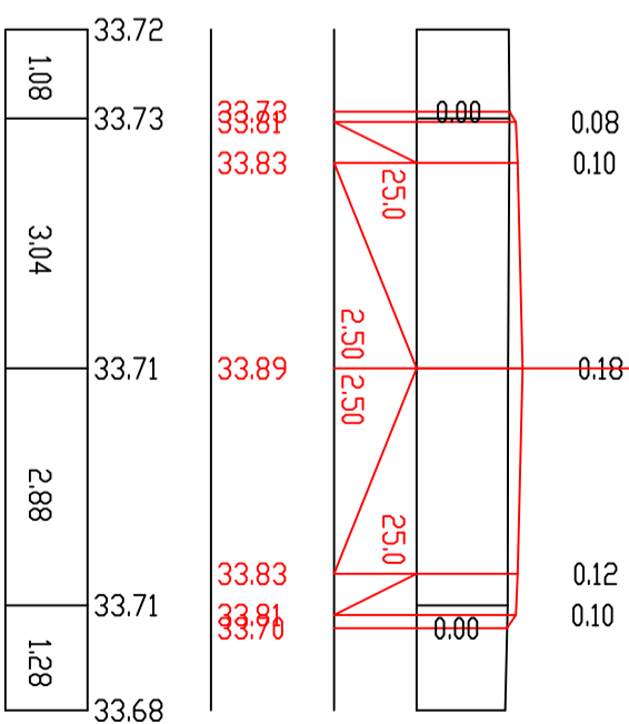
П-148 ПК 29+40.00
