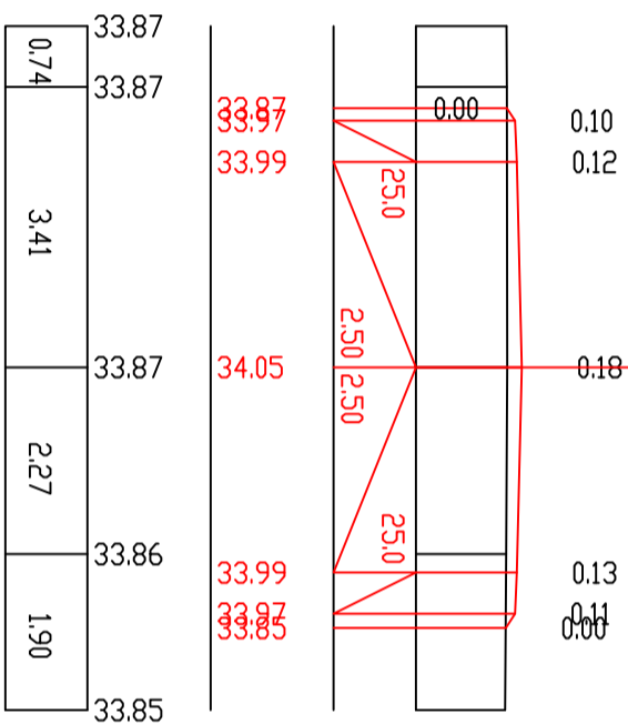
П-146 ПК 29+00.00
