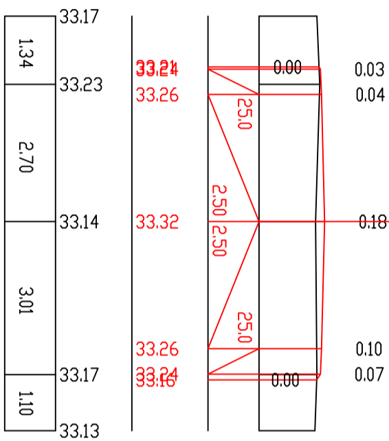
П-152 ПК 30+20.00
