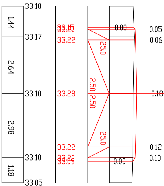
П-153 ПК 30+40.00
