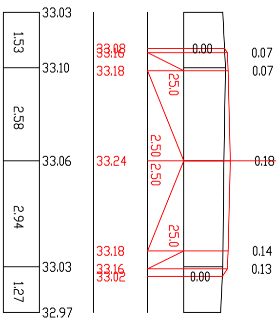
П-154 ПК 30+60.00
