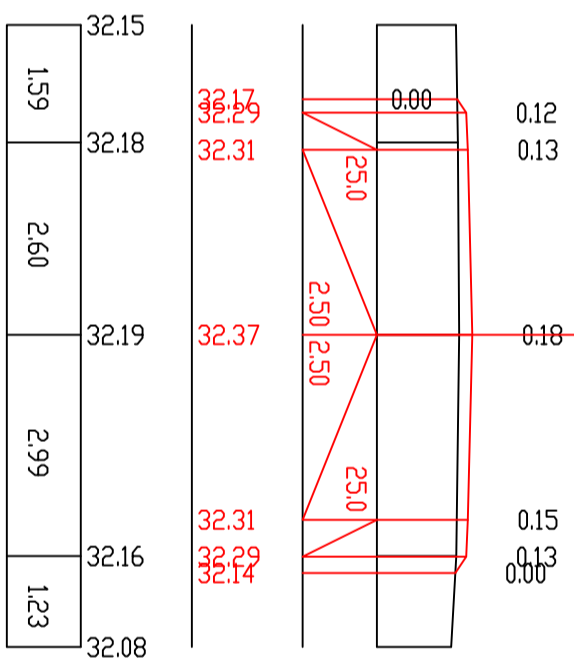
П-165 ПК 32+80.00
