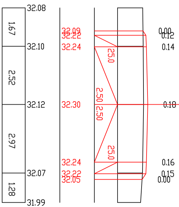
П-166 ПК 33+00.00
