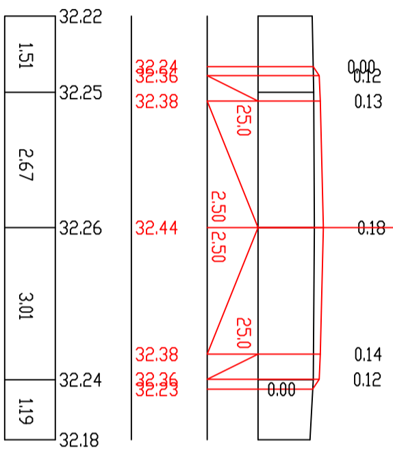
П-164 ПК 32+60.00
