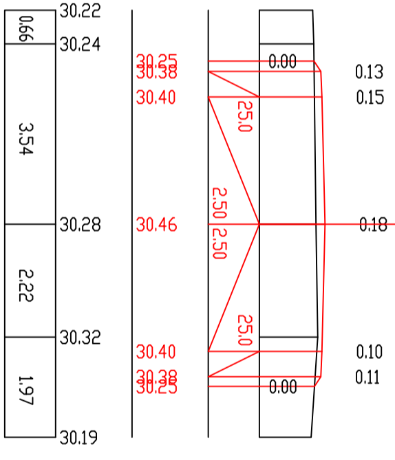
П-213 ПК 42+40.00
