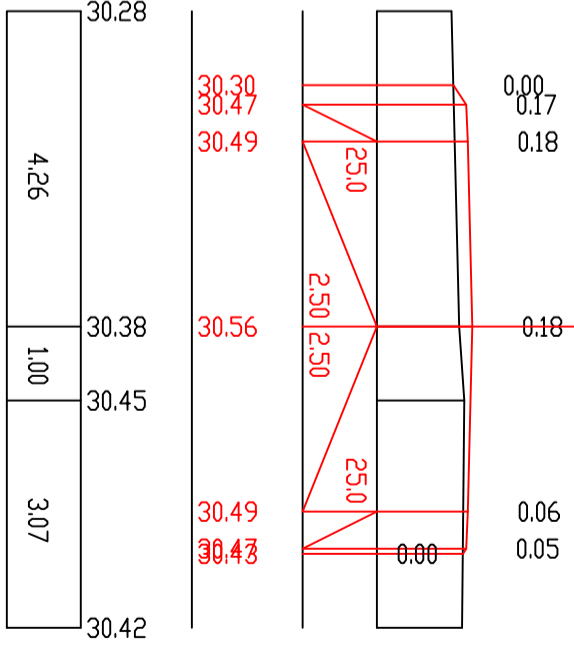
П-214 ПК 42+60.00
