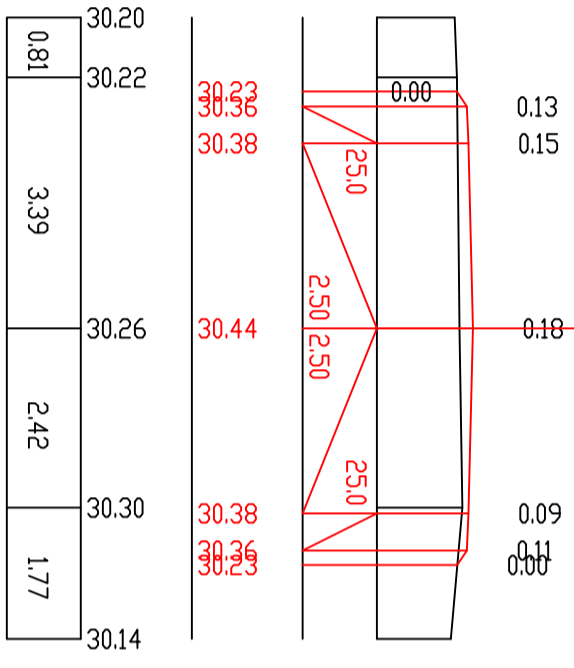
П-212 ПК 42+20.00
