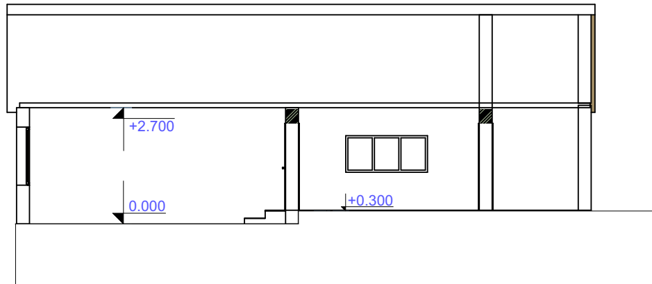
ჭრილი 1-1 მ 1:100
