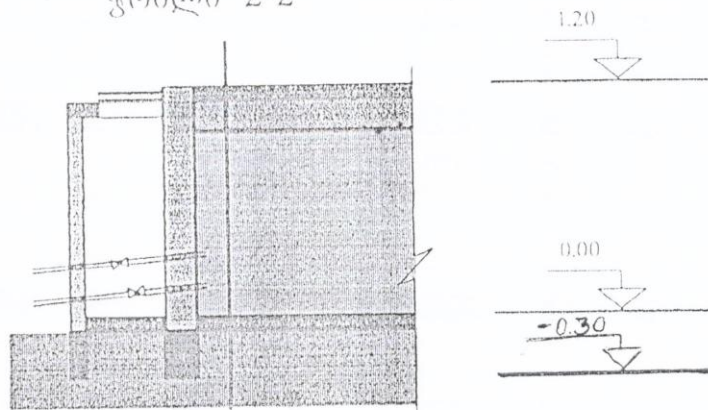
ჭრილი 2-2
