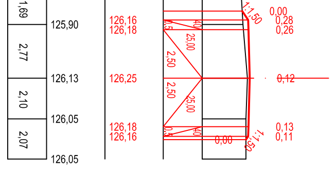
Г-26 ПК 9+50,00
