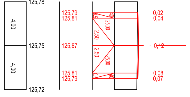
Г-24 ПК 8+50,00
