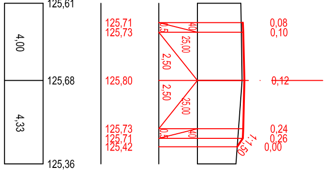
Г-21 ПК 7+00,00
