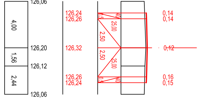
Г-27 ПК 10+00,00
