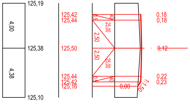
Г-20 ПК 6+50,00
