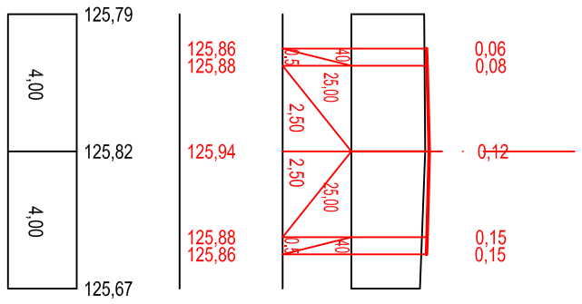
Г-22 ПК 7+50,00
