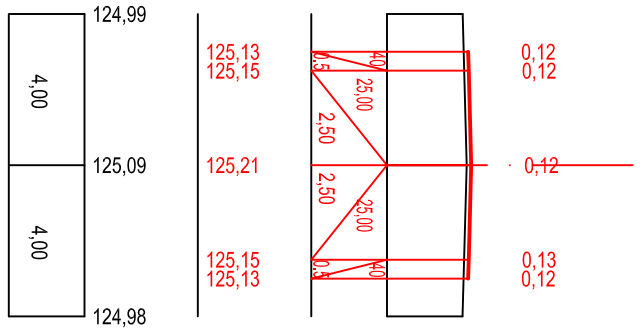
Г-19 ПК 6+00,00
