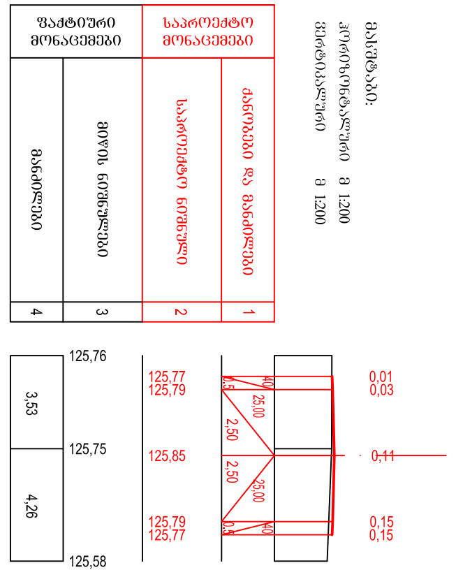
Г-23 ПК 8+00,00
