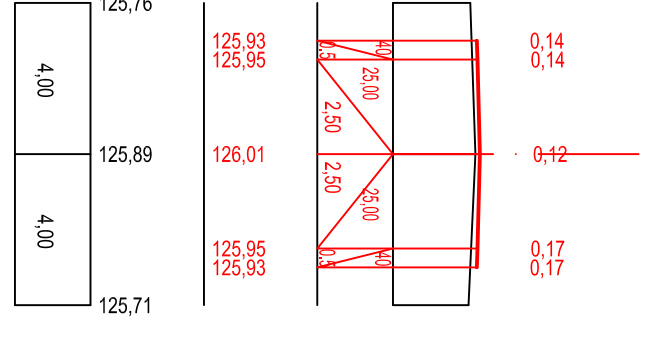
Г-25 ПК 9+00,00
