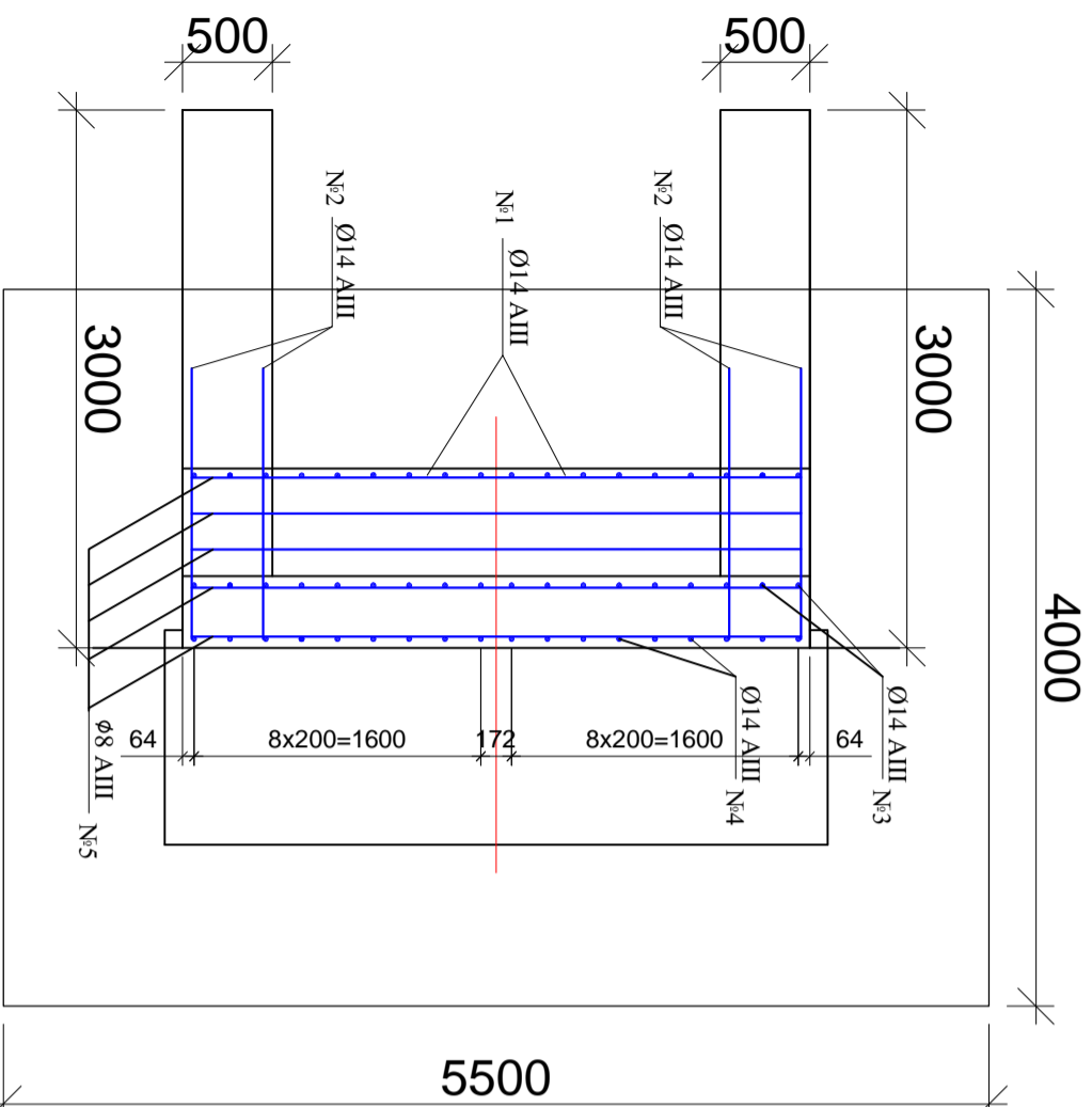
სანავიტირო გუნჯის საპირაღმოს კედლის არმირების აგოკრება და სპეციფიკაცია
