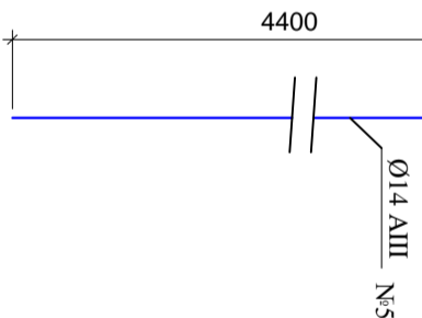
სანავიტირო გუნჯის საპირაღმოს კედლის არმირების აგოკრება და სპეციფიკაცია
