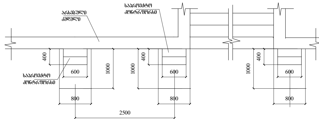
კონტრფორსების განლაგების გეგმა
