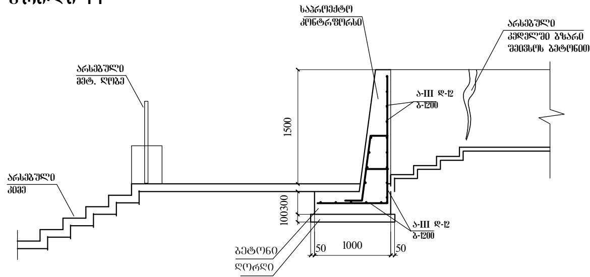
ჭრილი 1-1
