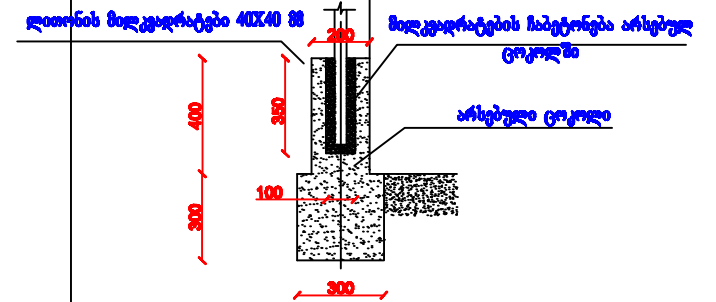
ჭრილი 1-1
