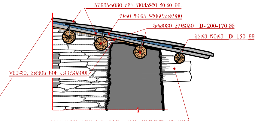
ჭრილი 2-2 ხაზი აღმოსავლეთით მ-1:100
