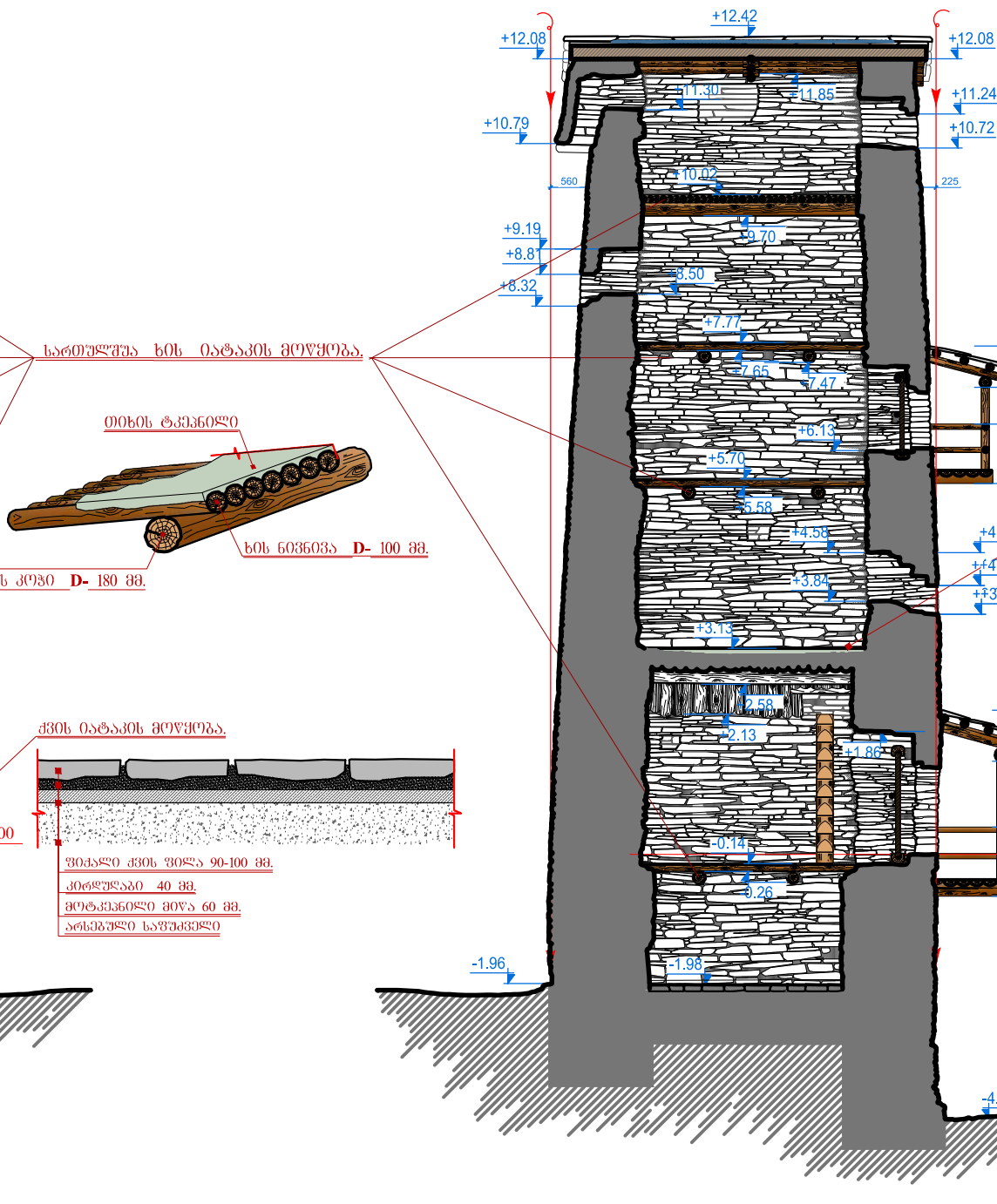
ჭრილი 4-4 ხალი სამხრეთით 1:100
