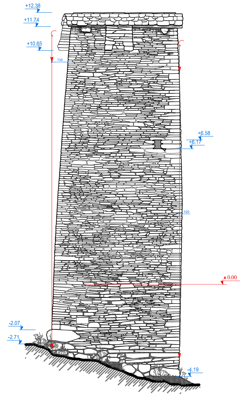
ჩრდილოეთი ფასადი 8-1:100
