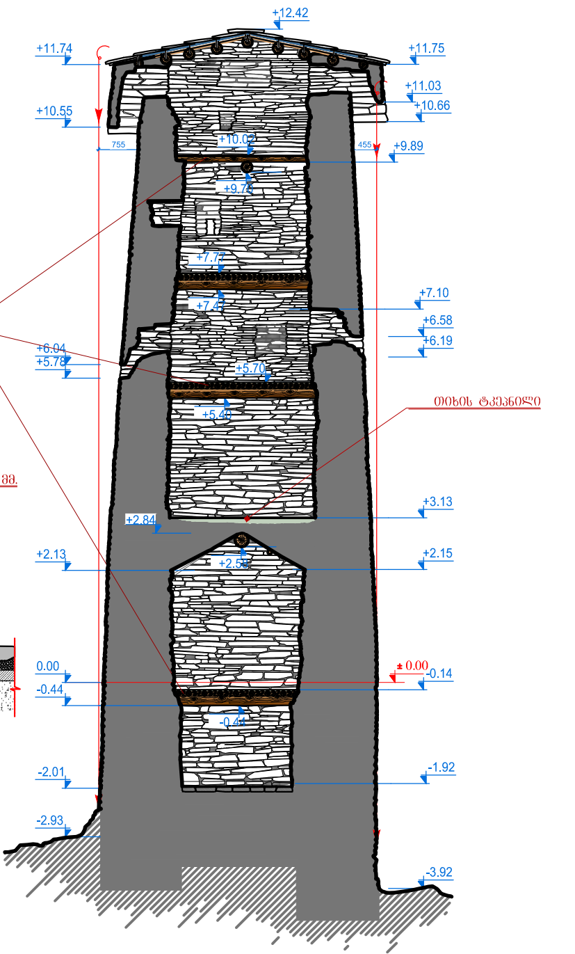
ჭრილი 2-2 ხაზი აღმოსავლეთით მ-1:100
