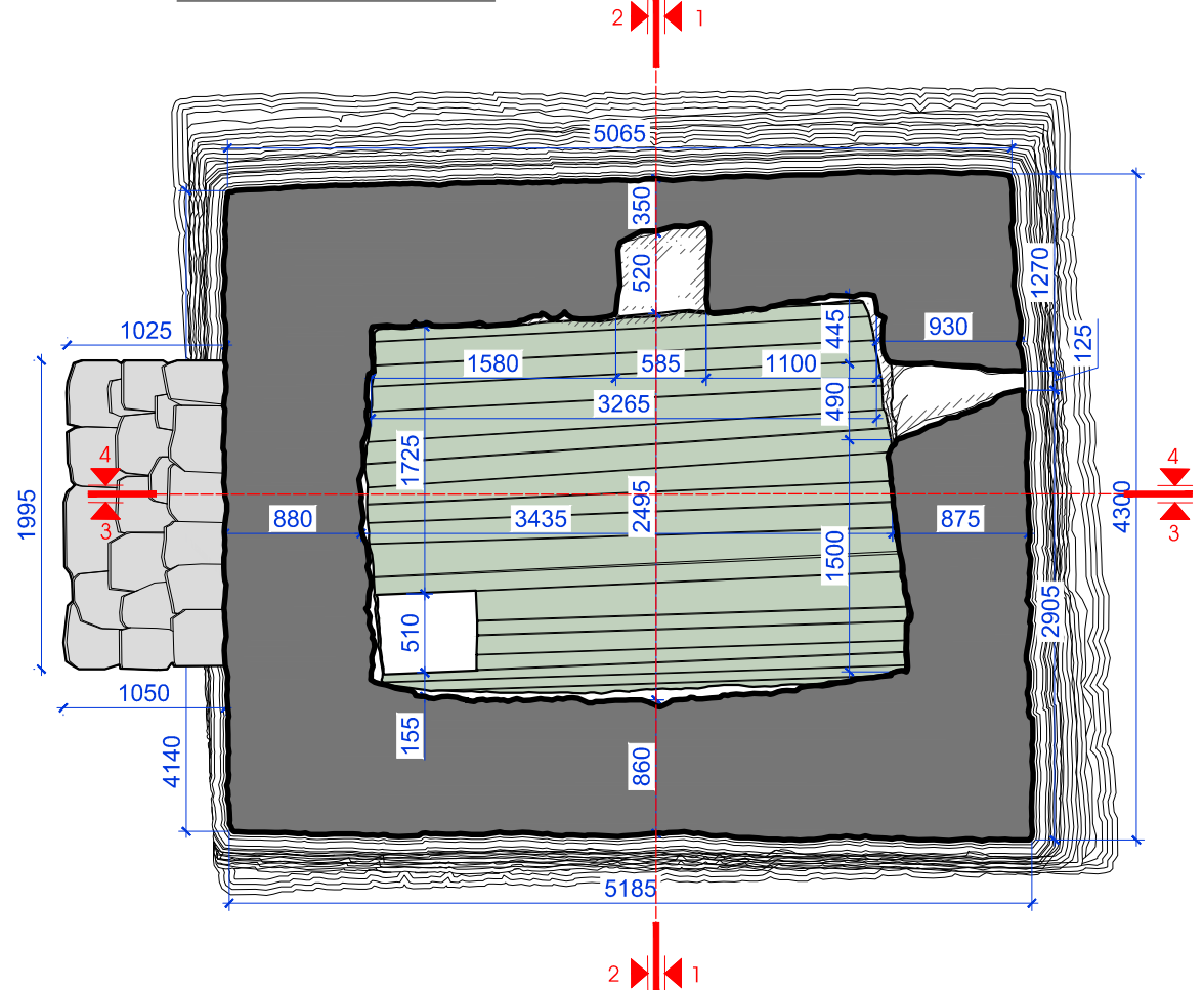
გეგმა +8,80 ნიშნულზე
