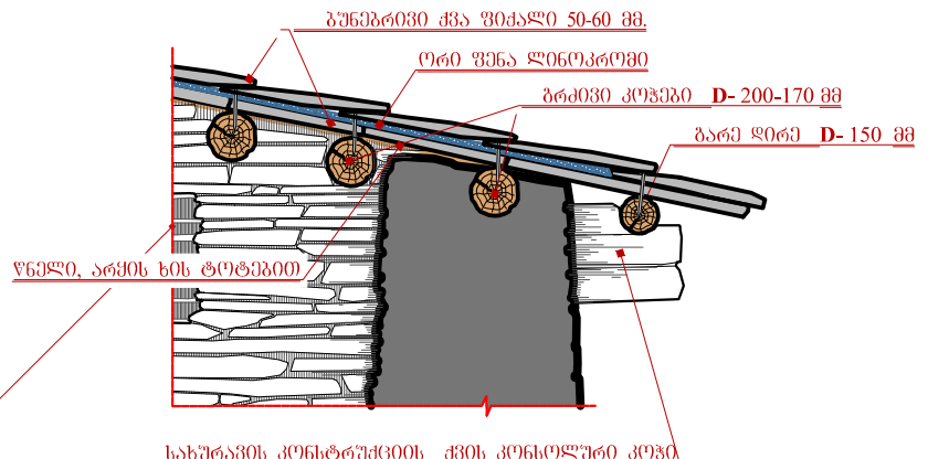
ჭრილი 4-4 ხალი სამხრეთით 1:100
