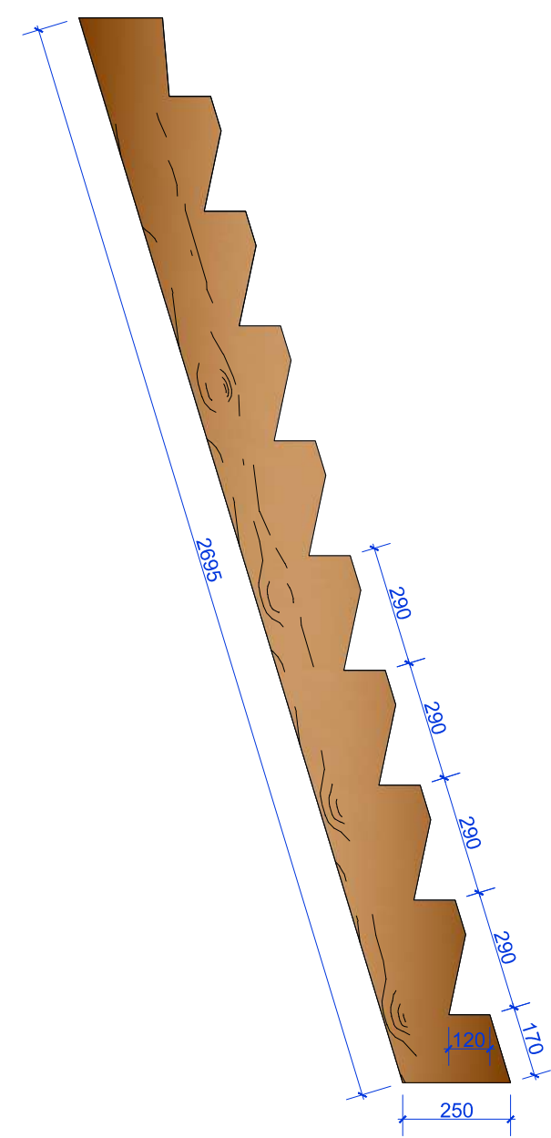
კვების მოწყობა ხის გორბით D-250 მმ.
