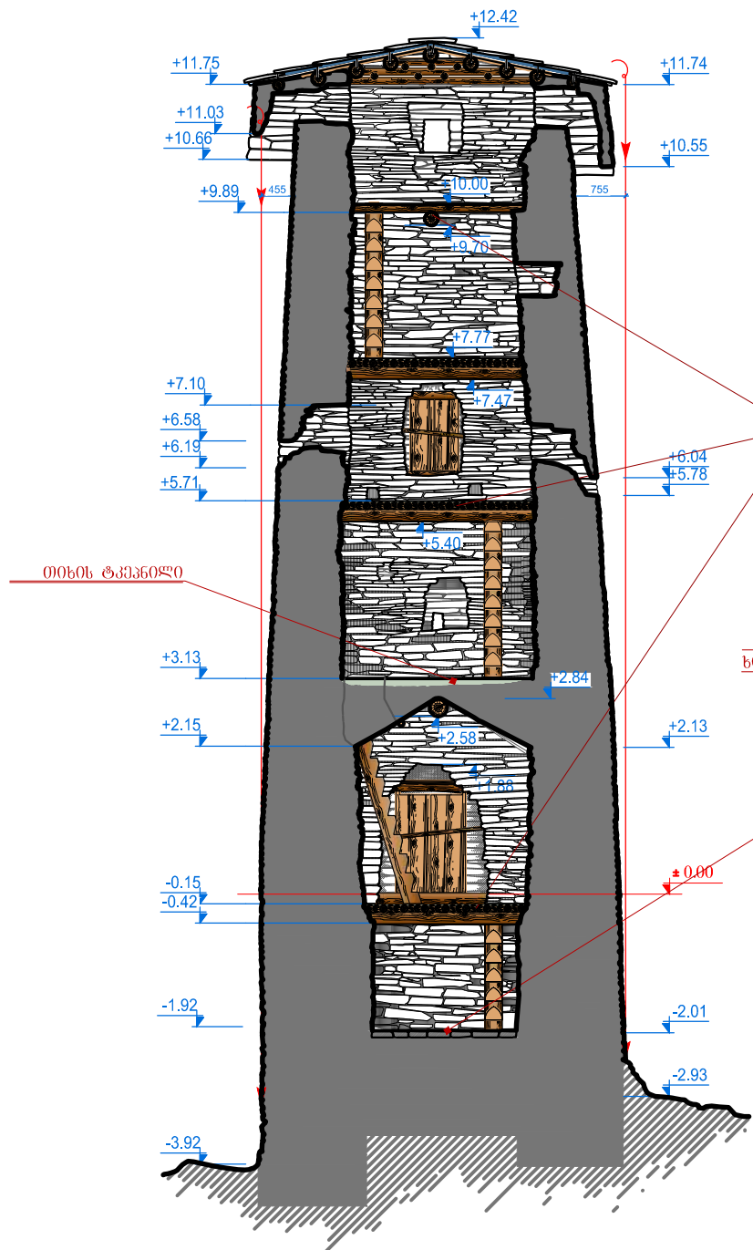
ჭრილი 1-1 ხაზი დასავლეთით მ-1:100
