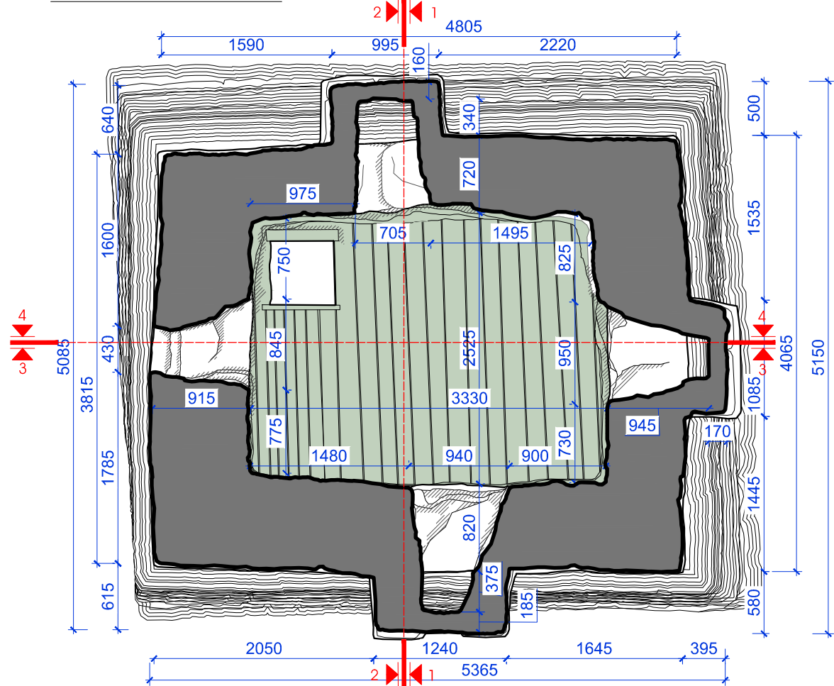
სახურავის გეგმა (ქვიშობა)
