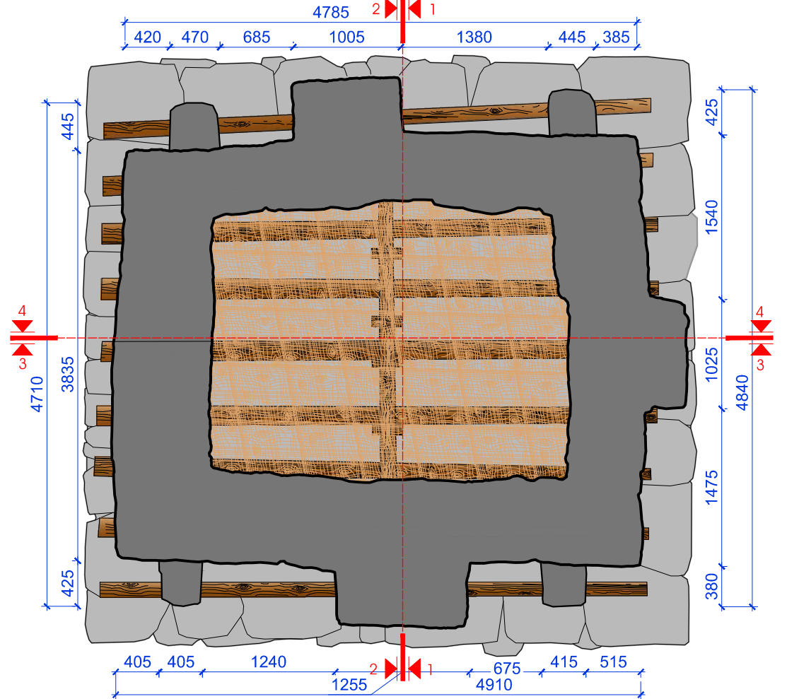
სახურავის გეგმა (ქვიშობა)
