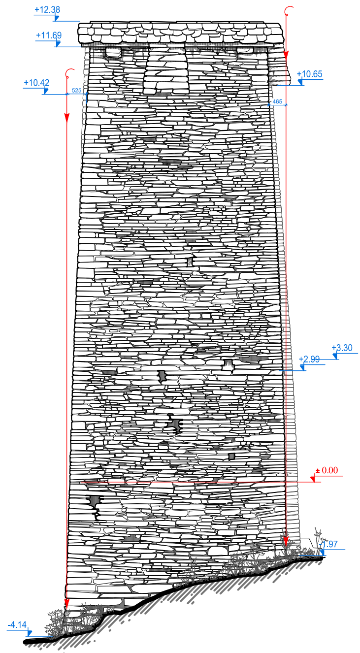
სამხრეთი ფასადი 8-1:100
