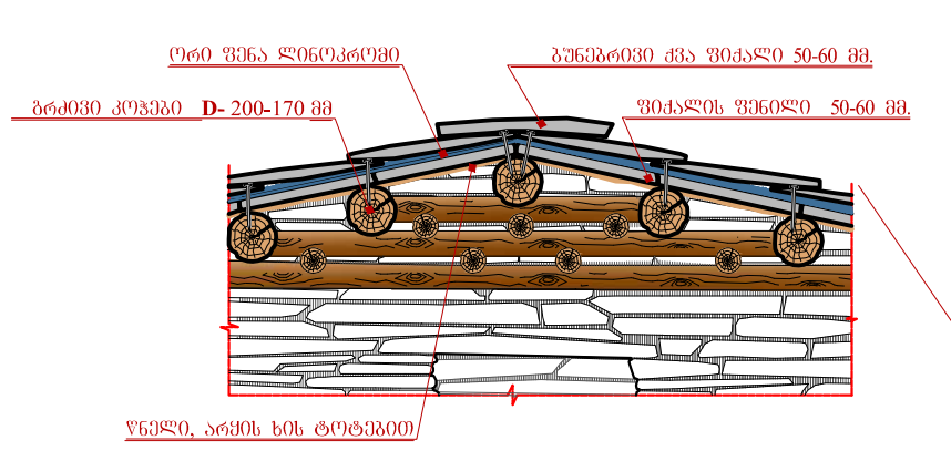
ჭრილი 3-3 ხალი ჩრდილოეთით 1:100
