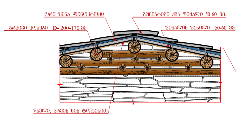
ჭრილი 1-1 ხაზი დასავლეთით მ-1:100
