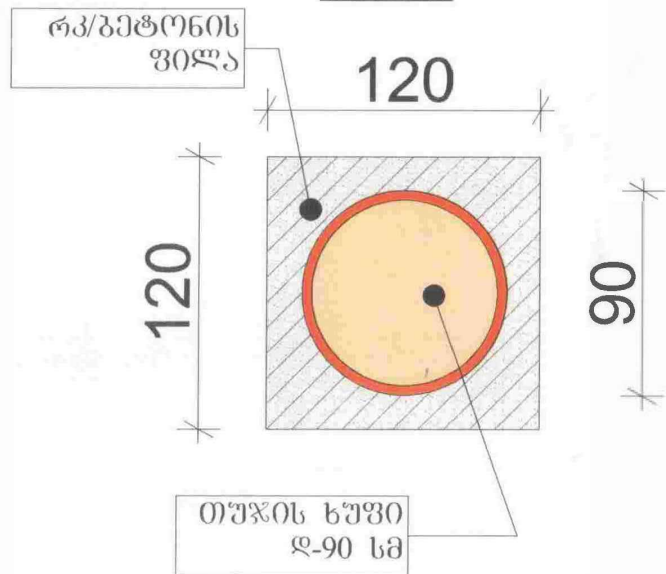
ჭის გადახურვა თუჯის ხუვით
