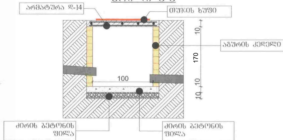
საკანალიზაციო ჭის ჭრილი ა-ა
