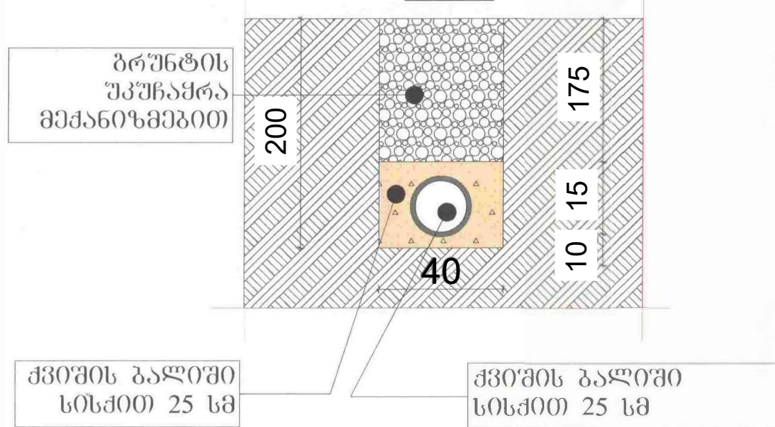
საკანალიზაციო მილის კვანძი
