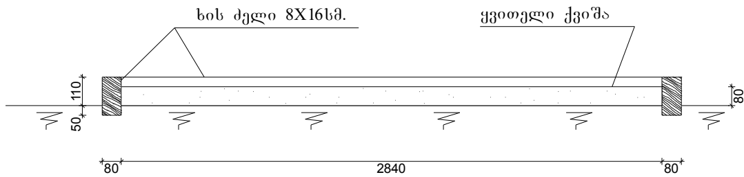
ჭრილი 1-1
