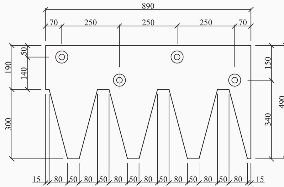
№2 ფოლადის ფურცელი δ=50
