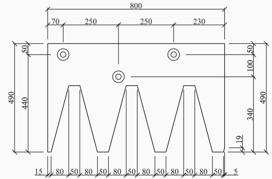
№3 ფოლადის ფურცელი δ=50
