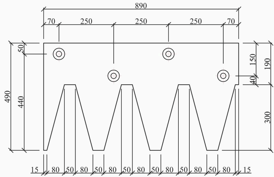
№4 ფოლადის ფურცელი δ=50
