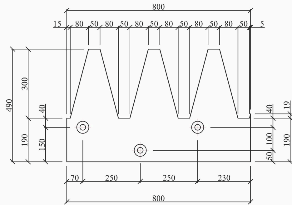
№4 ფოლადის ფურცელი δ=50
