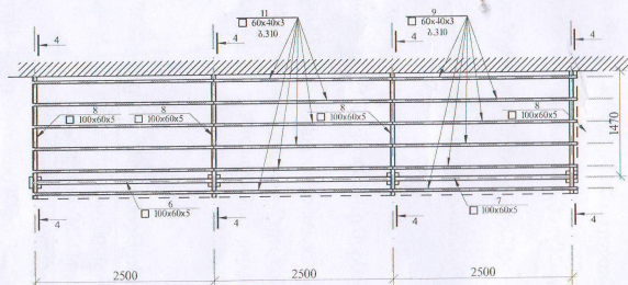
სანთრავის მოწყობის გეგმა მ. 1:50
